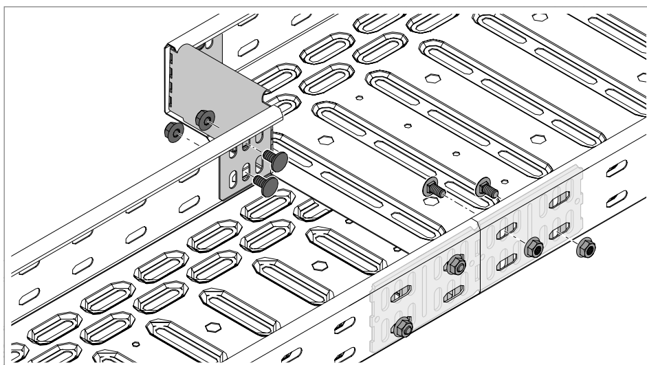
Afb. 74: Koppel- en hoekverbinder en reduceerhoek
