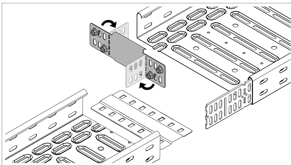
Afb. 73: Reduceerhoek buigen
