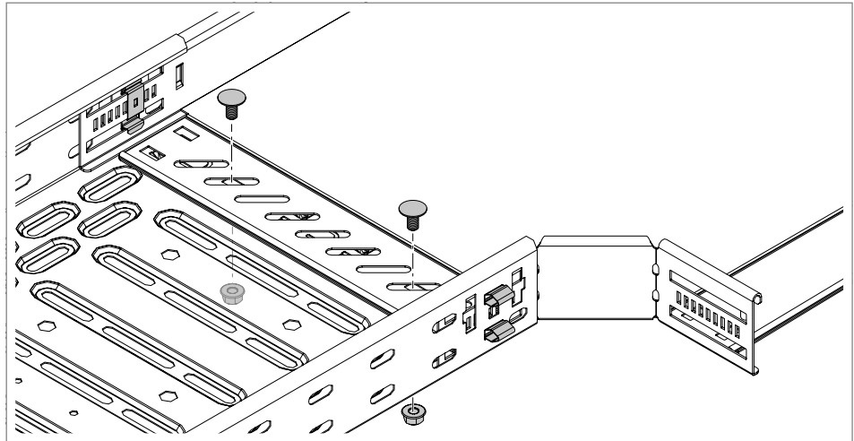
Afb. 47: Voegplaat vastschroeven
