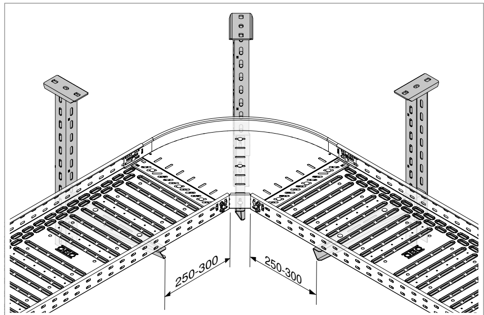
Afb. 44: Voorbeeld ondersteuning hulpstuk 90° bocht 400 mm breedte
