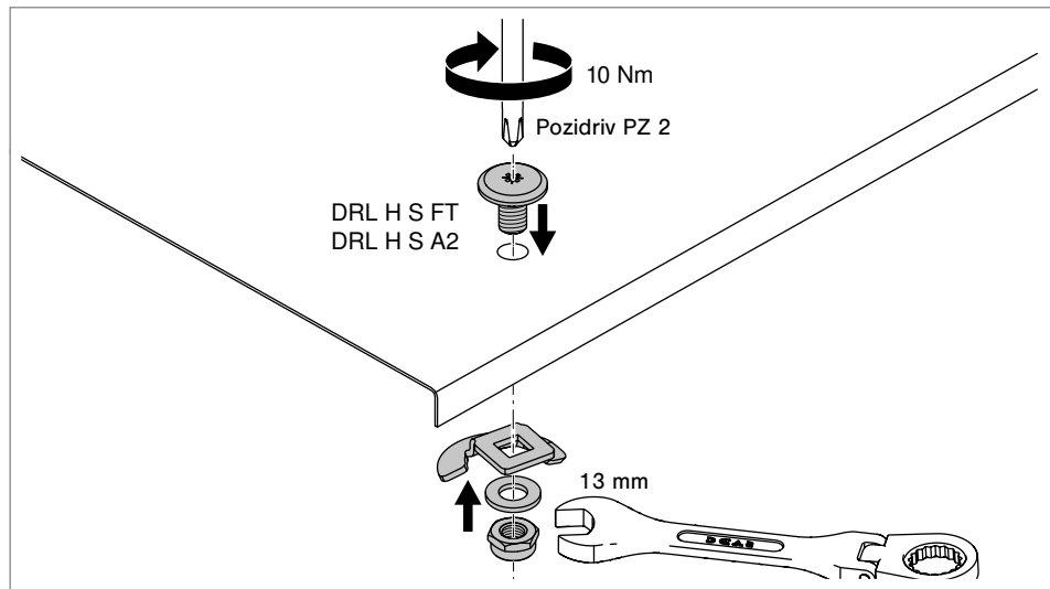
Afb. 87: Draaigrendel schroeven
