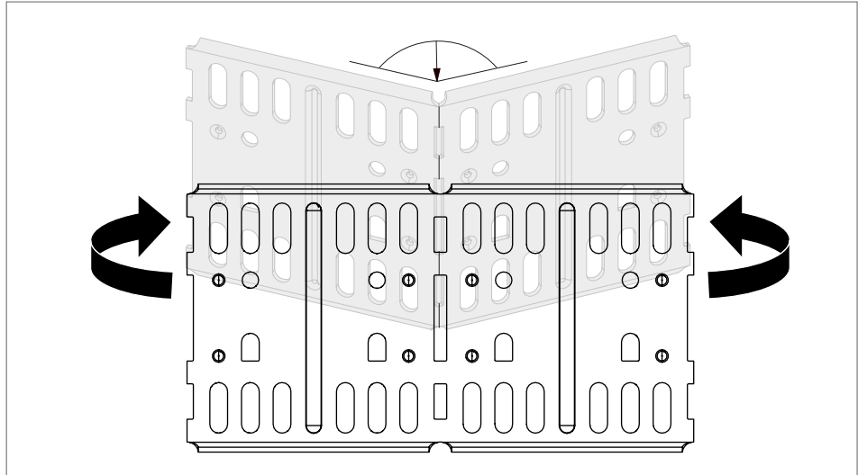
Afb. 31: Koppel- en hoekverbinder RLVL buigen
