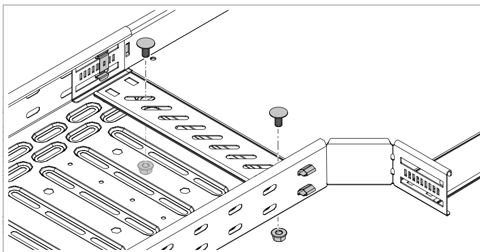
Afb. 52: Voegplaat vastschroeven
