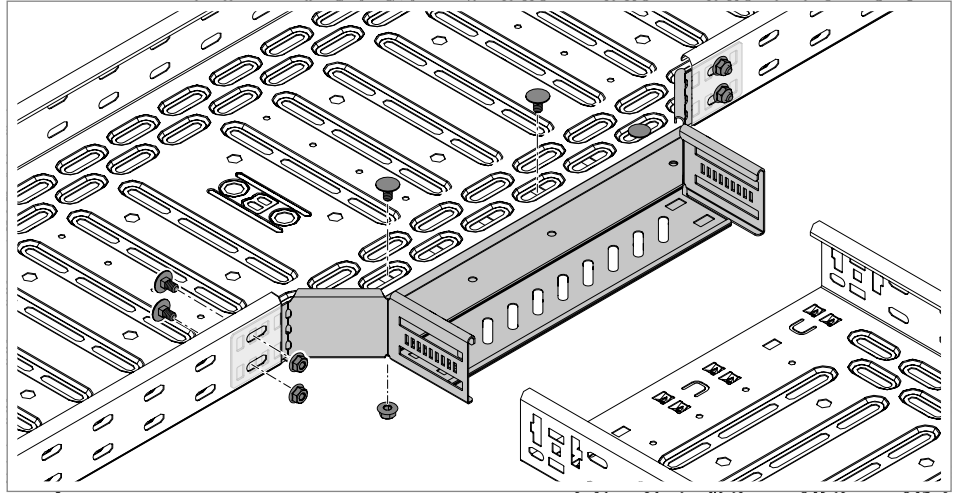
Afb. 56: Aanbouw T-stuk op doorgaande kabelgoot schroeven
