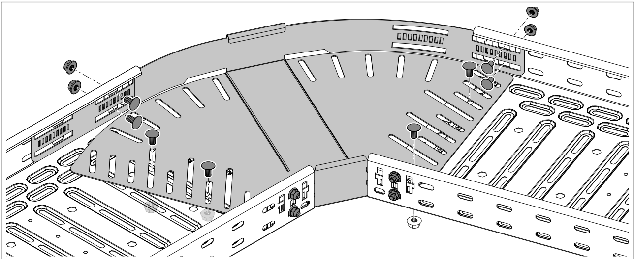
Abb. 66: Verbinders en voegplaten op de goten schroeven
