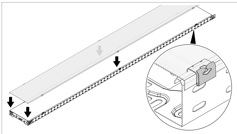
Afb. 85: Deksel opklikken
