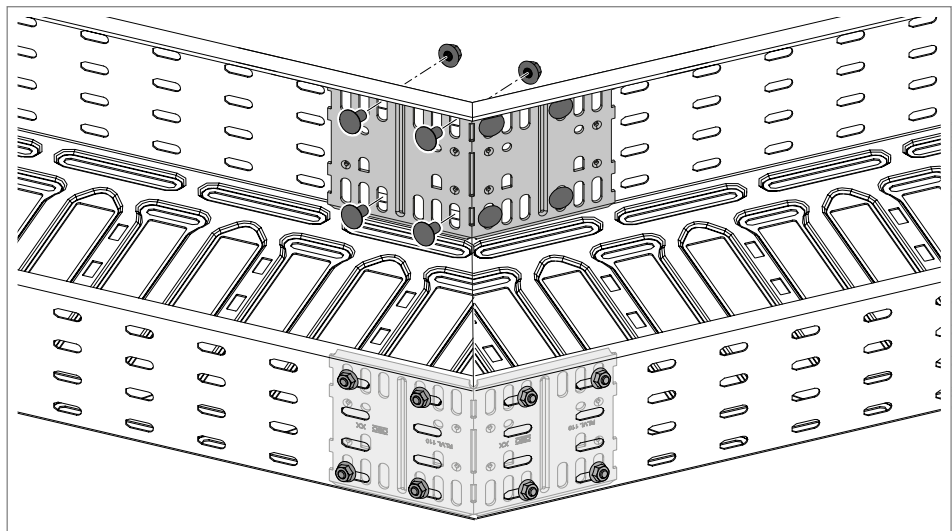
Afb. 32: Koppel- en hoekverbinder RLVL vastschroeven
