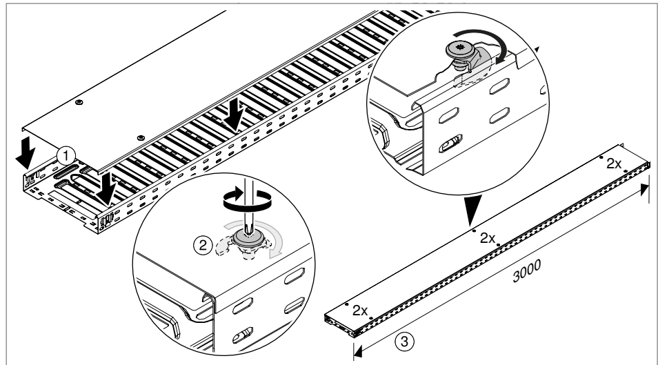
Afb. 89: Deksel met draaigrendel monteren
